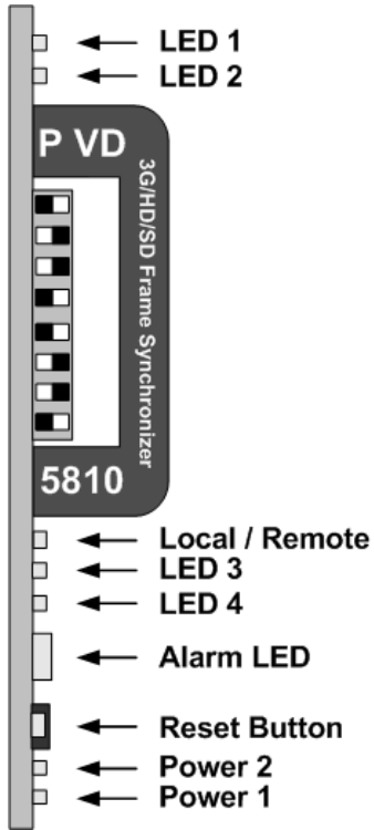
Figure 5: Card Edge
